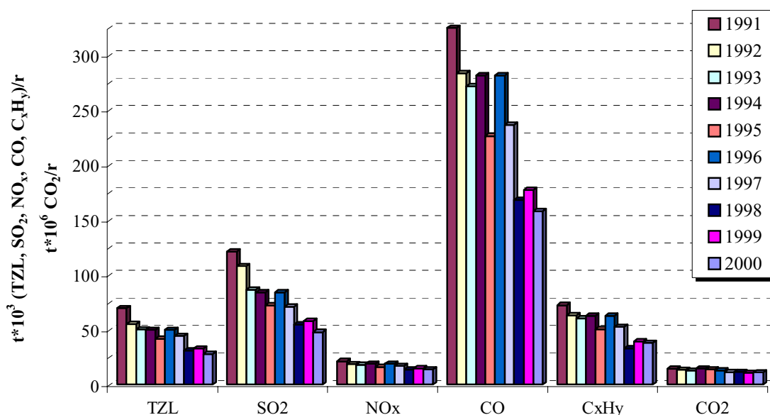
OBR. 5.2 MNOŽSTVÍ PRODUKOVANÝCH EMISÍ REZZO3 (1991-2000)
